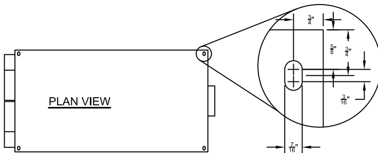
HANGER ROD LOTS 4PL. TYP.
